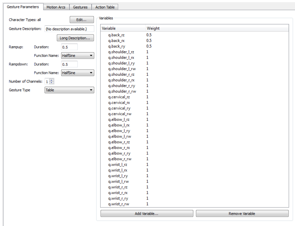
Figure 8-3. Gesture Parameters Tab
