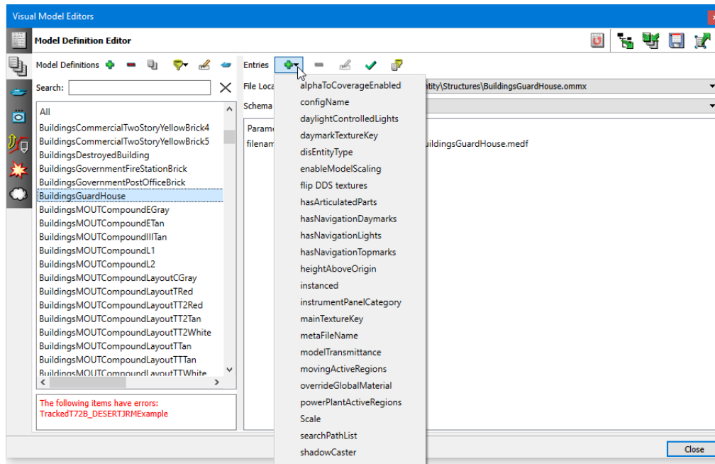
Figure 14-4. Add parameter list
