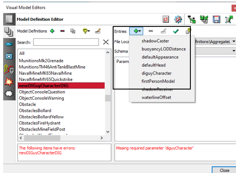
Figure 23-3. Add parameter list
