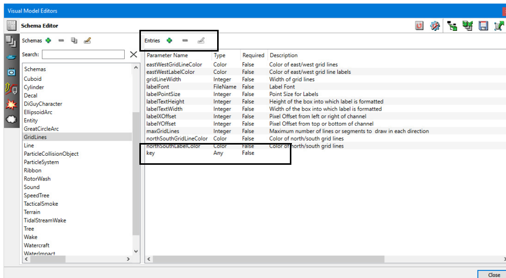
Figure 13-3. New schema parameter
