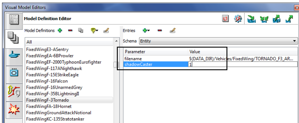
Figure 6-8. Editable parameter
